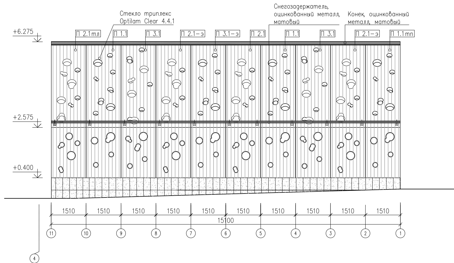
ФАСАД В ОСЯХ 11-1
