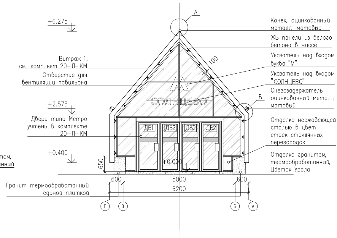
ФАСАД В ОСЯХ 011-01
