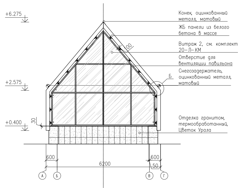
ФАСАД В ОСЯХ 011-01
